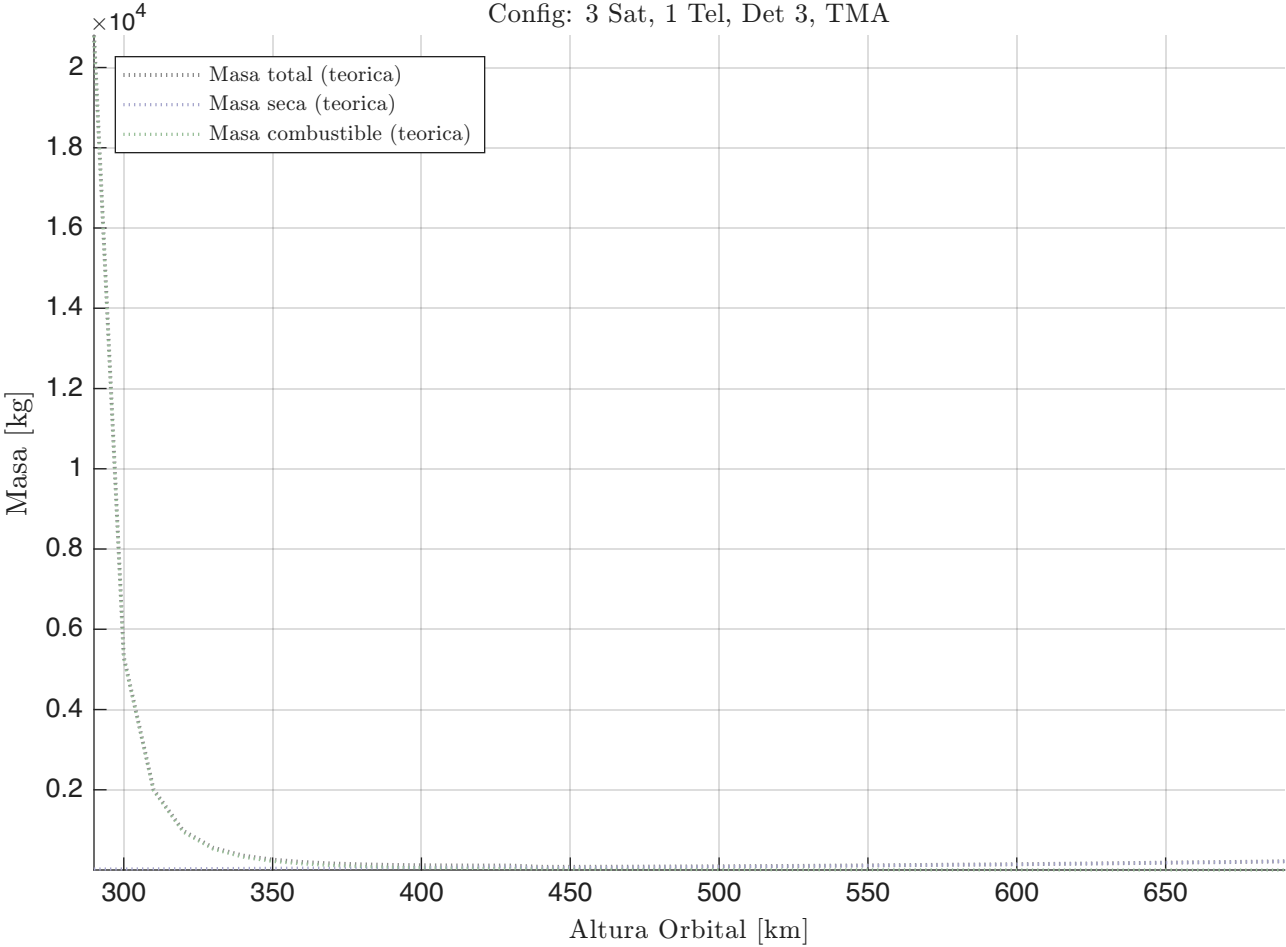
Desglose de Masas vs. Altura Config: 3 Sat, 1 Tel, Det 3, TMA
